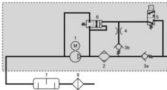
Luftversorgungsaggregat
